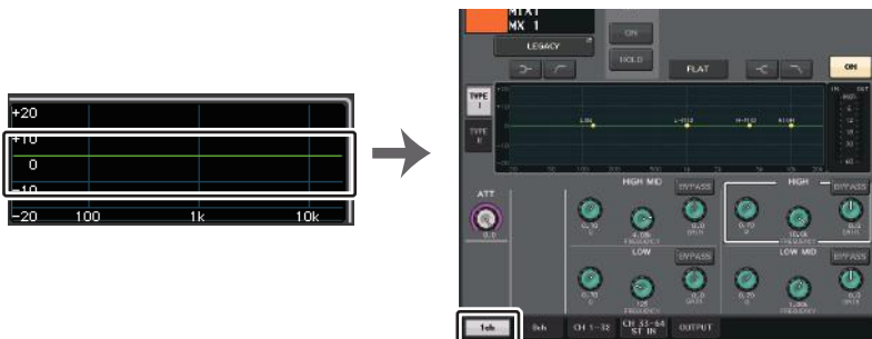
Экран SELECTED CHANNEL VIEW (Представление выбранного канала)
